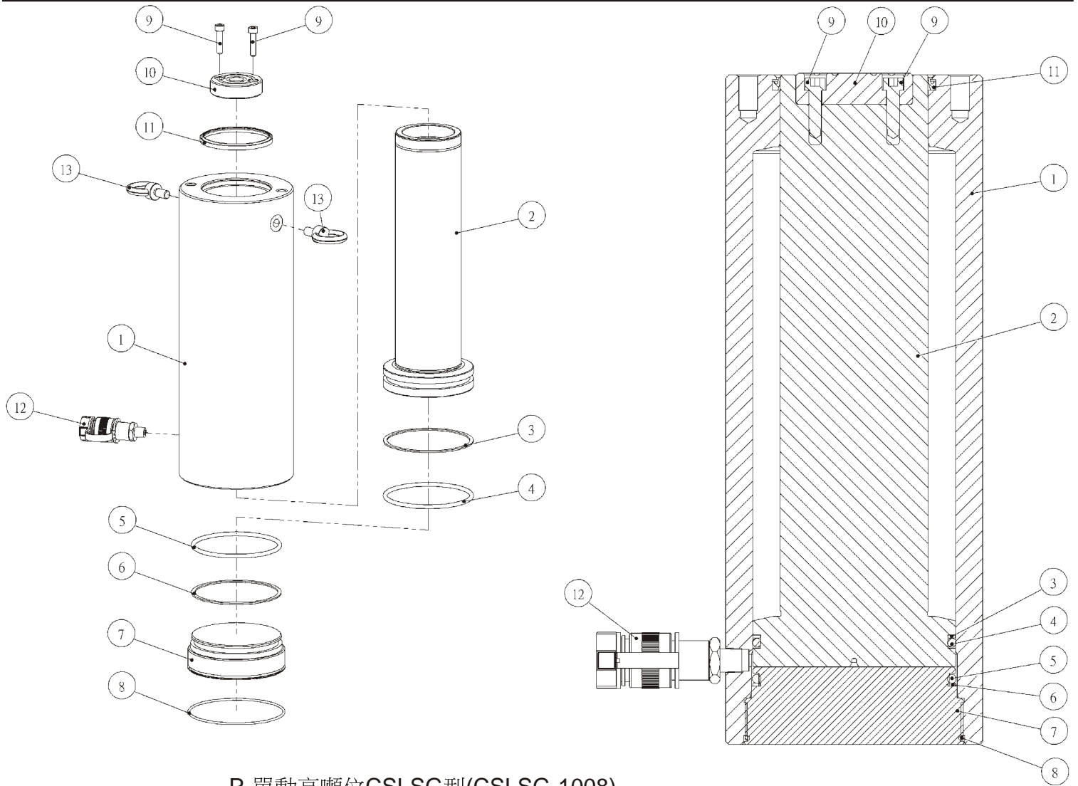
P-單動高噸位CSLSG型(CSLSG-1008)
