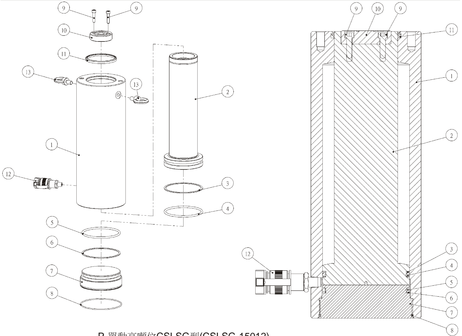
P-單動高噸位CSLSG型(CSLSG-15012)
