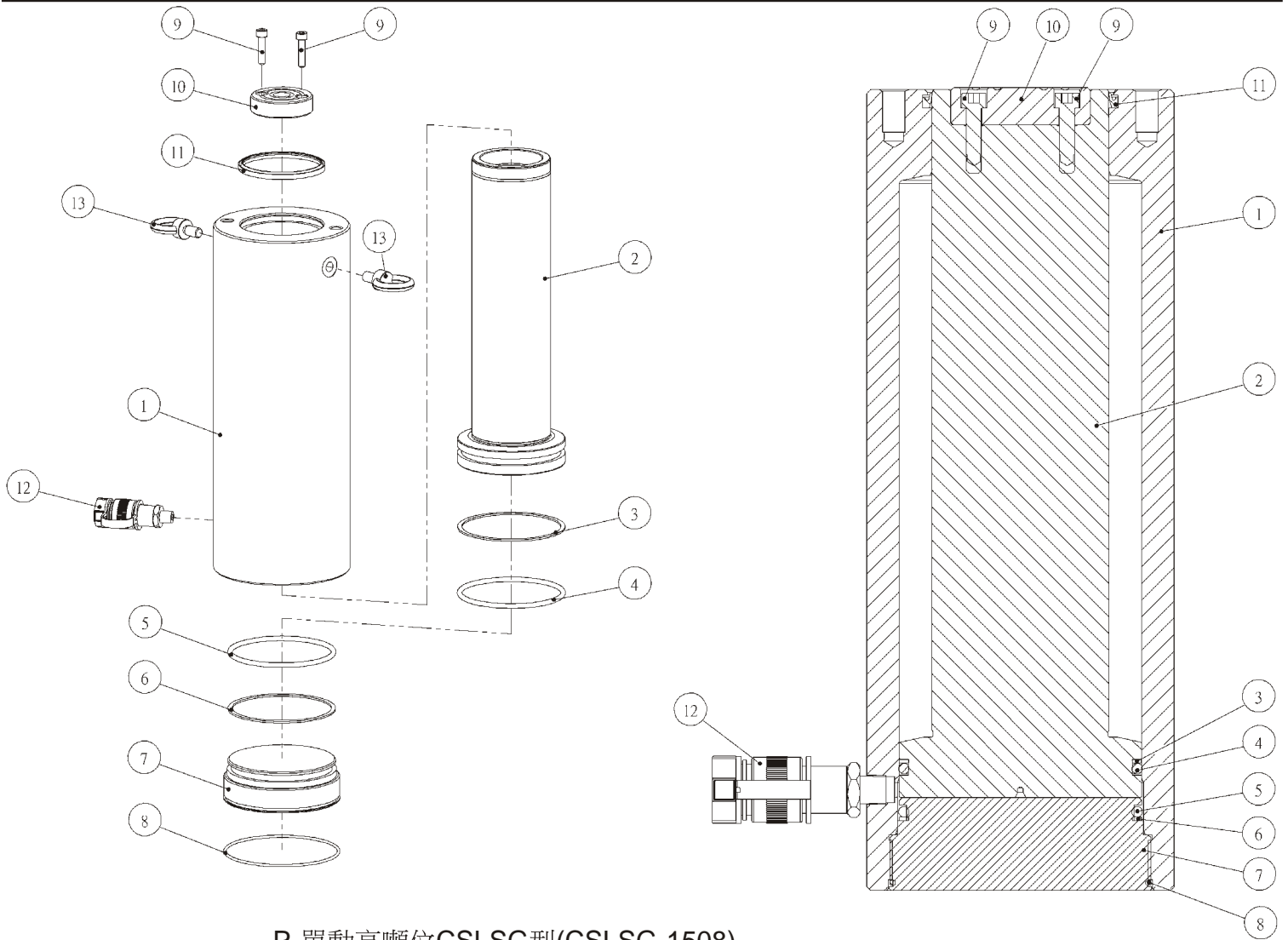
P-單動高噸位CSLSG型(CSLSG-1508)
