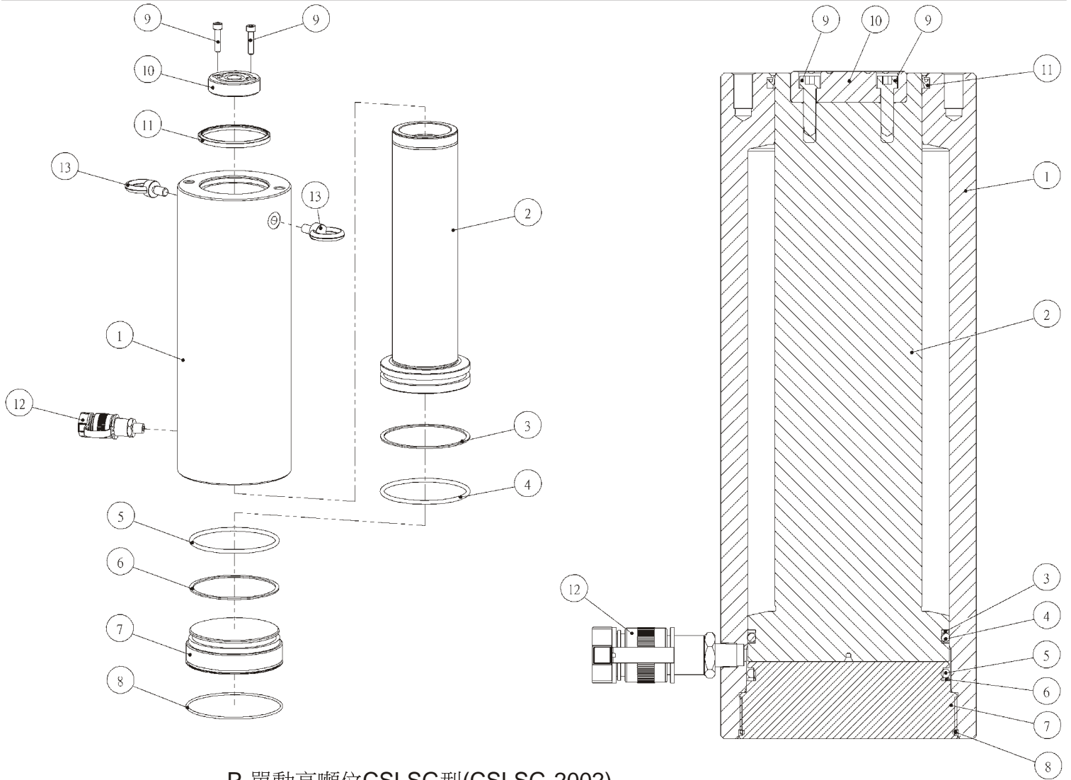
P-單動高噸位CSLSG型(CSLSG-2002)
