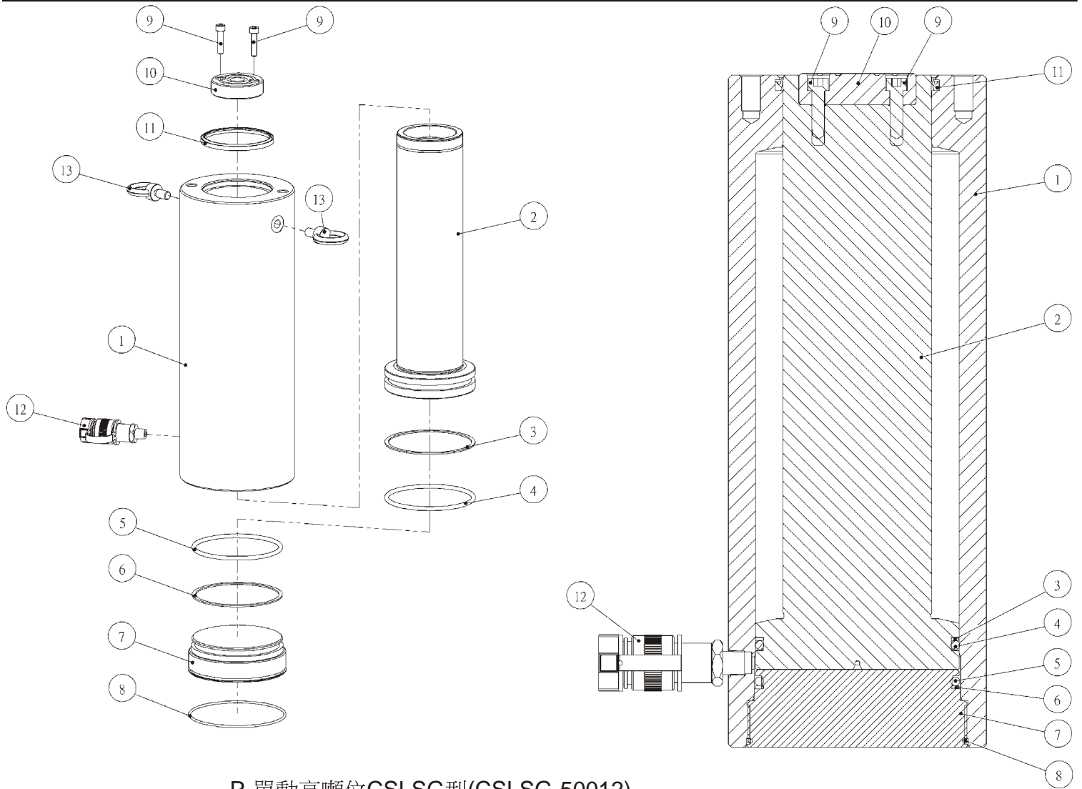
P-單動高噸位CSLSG型(CSLSG-50012)
