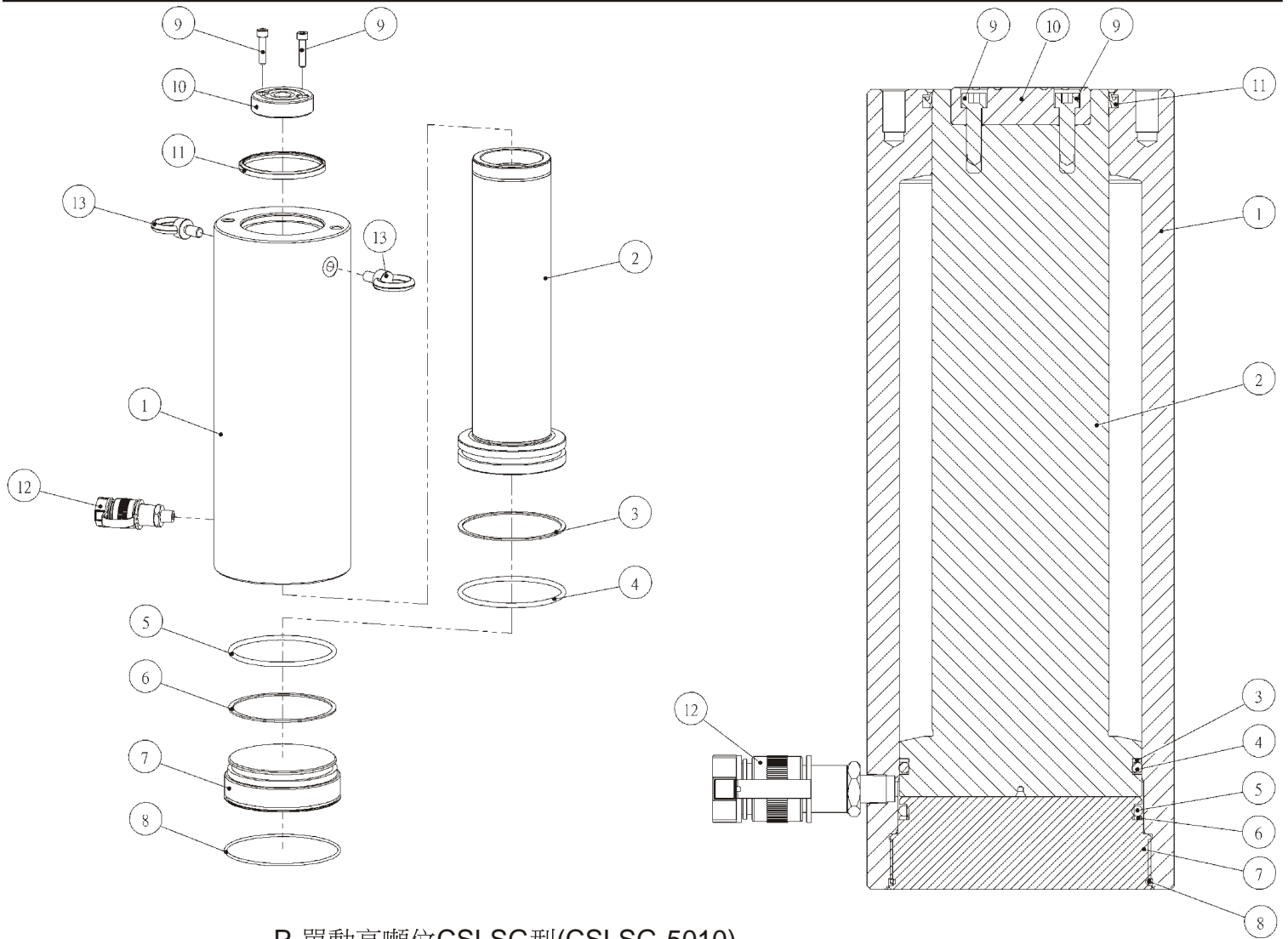
P-單動高噸位CSLSG型(CSLSG-5010)
