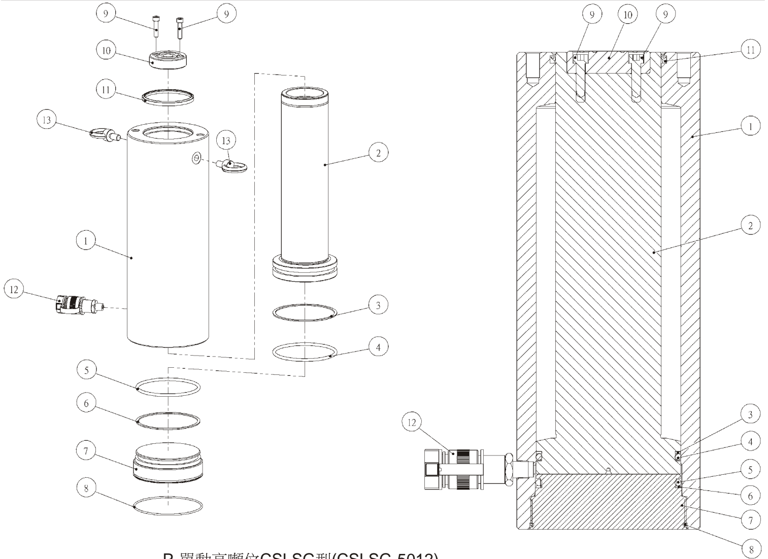
P-單動高噸位CSLSG型(CSLSG-5012)
