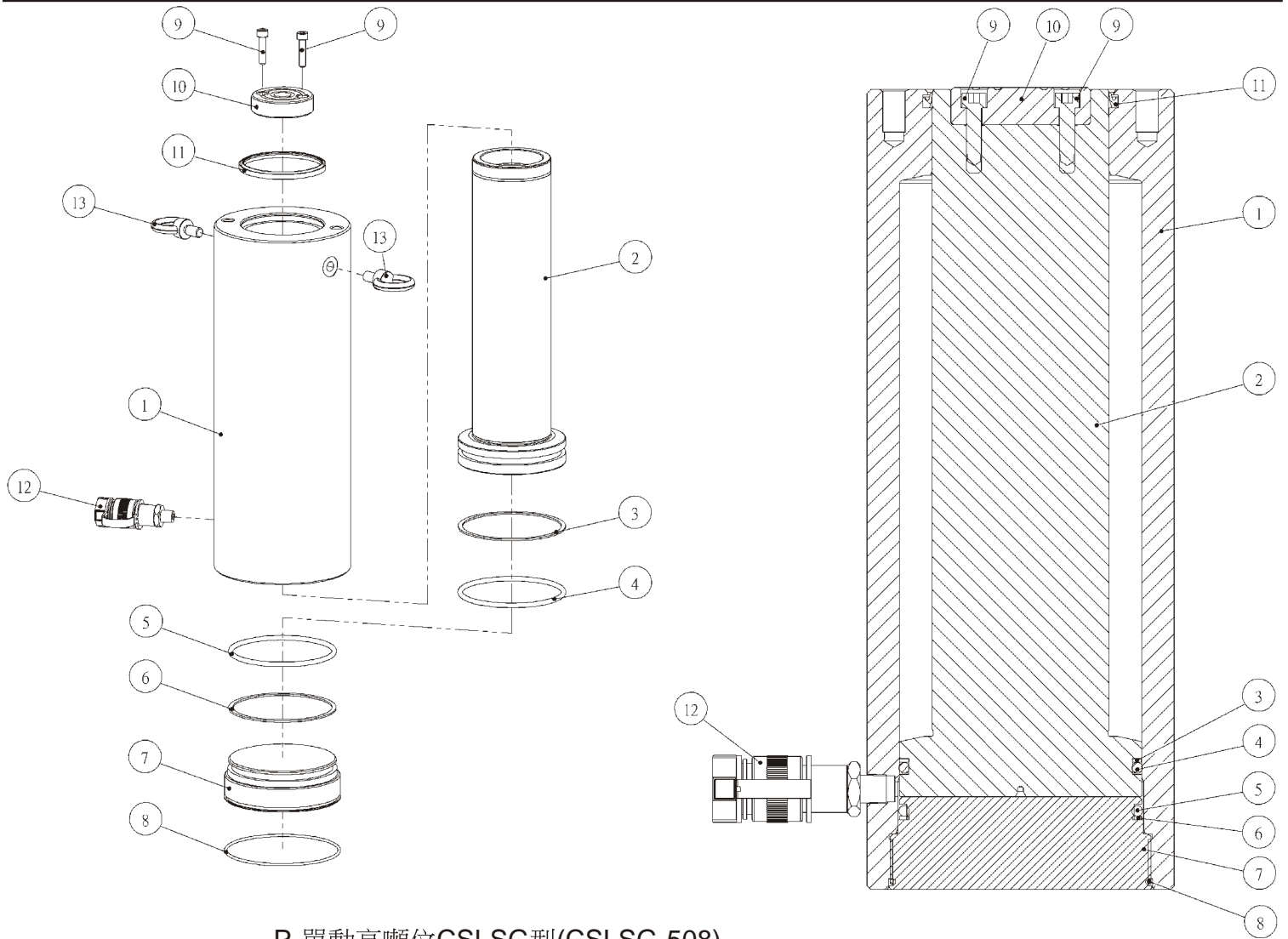
P-單動高噸位CSLSG型(CSLSG-508)
