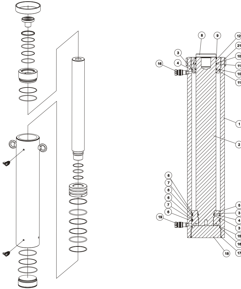
M-雙動/塞底/主軸內牙/上螺帽/溝槽墊塊型(RSR-20036)
