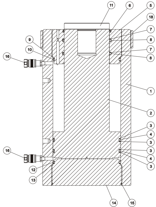
M1-雙動/塞底/主軸內牙/上螺帽/溝槽墊塊型 (RSR-50024)
